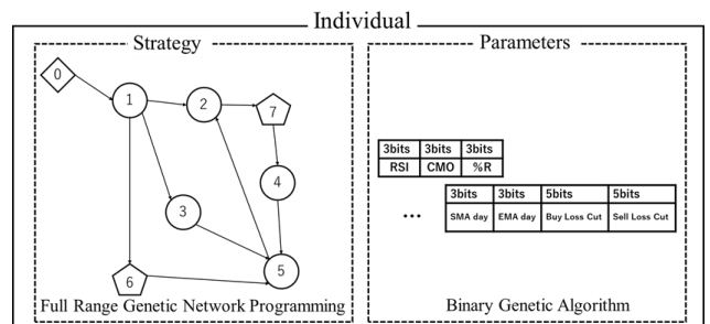
図5 提案モデルの個体例
