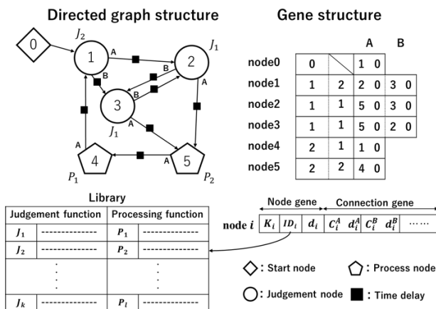
図1 GNPの基本構造
