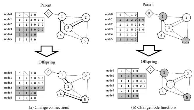
図3 GNPの突然変異
