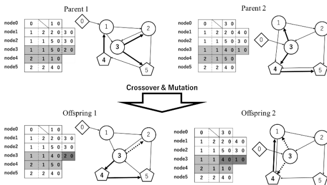
図4 FRGNPの進化操作
