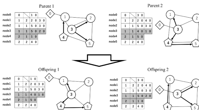
図2 GNPの交叉
