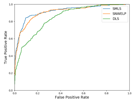
図 2: 各モデルにおける ROC 曲線の比較
