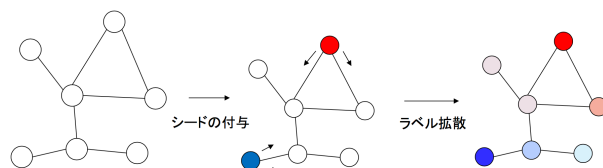
図 1: ラベル拡散法の概要
